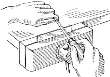
Fig. 92B —Turning the Edge
