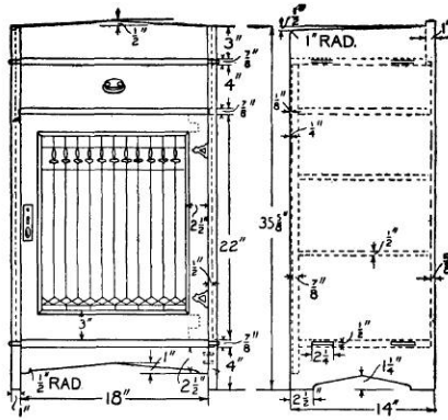
Fig. 112—Cabinet Details
