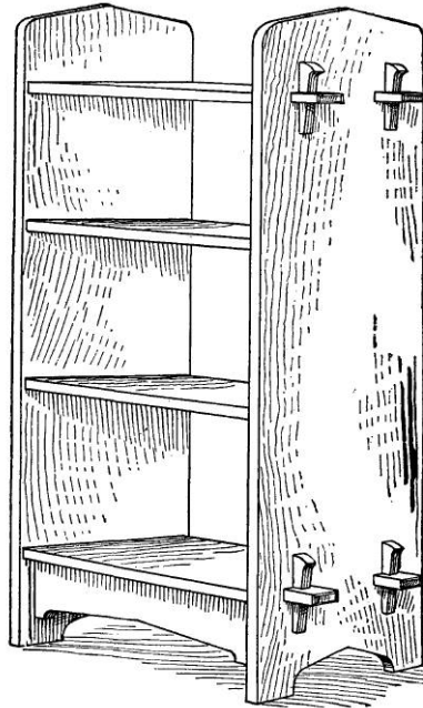
Fig. 93—Magazine Stand
